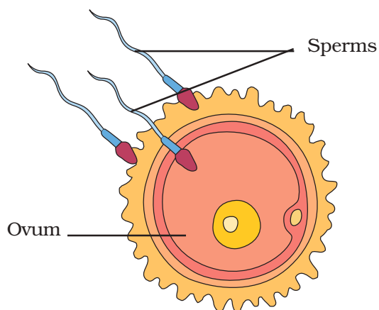
Fig. 9.5 : Fertilisation
